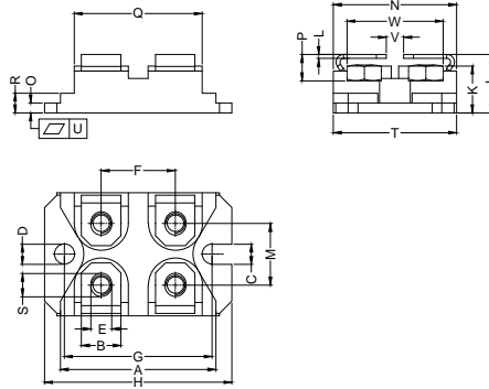
Dimensions SOT -227
